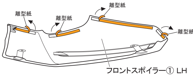
図 11 裏面視 ※LH図示 左右共通作業
