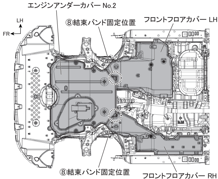
図 10 下面視
