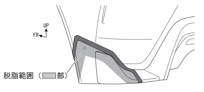
図8 ※LH図示 左右共通作業
