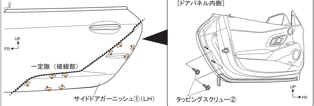
図10 ※LH図示 左右共通作業
