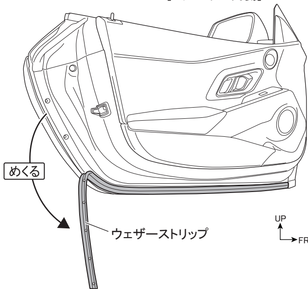
図2 ※LH図示 左右共通作業 [ドアパネル内側]
