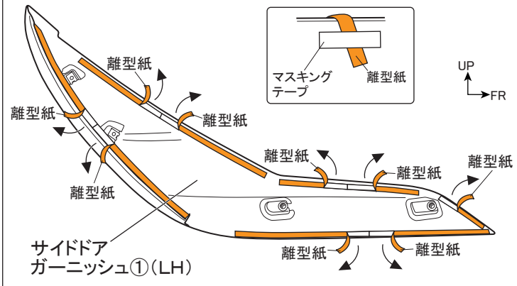
図9 裏面視 ※LH図示 左右共通作業
