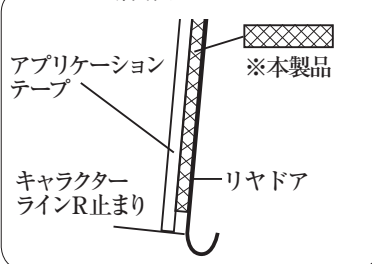
A-A 断面図
