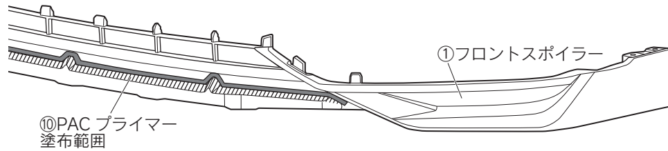
図 14 ※LH図示 左右共通作業
