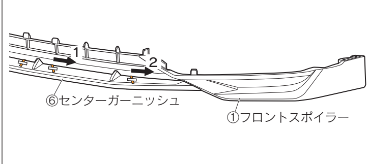
図 18 下面視 ※LH図示 左右共通作業
