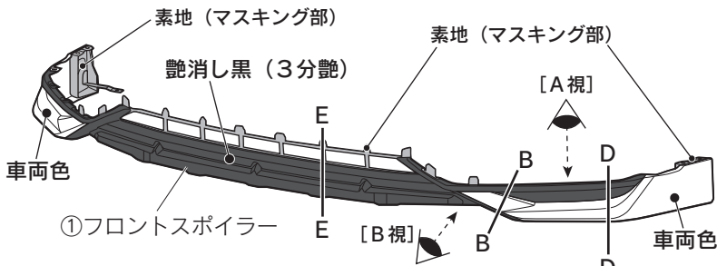
図 10 ※LH 図示 左右共通作業
