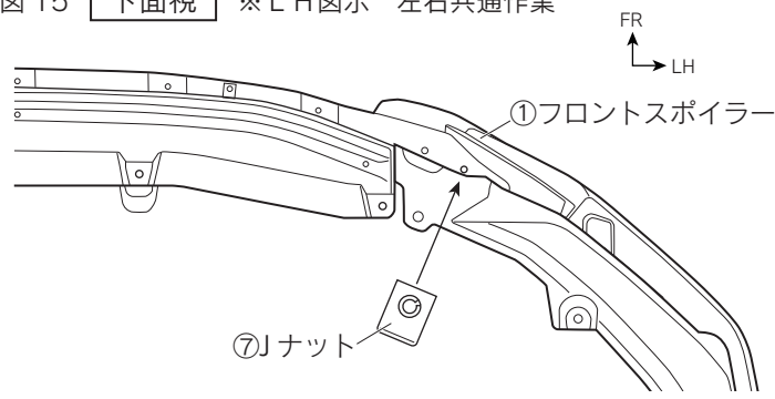
図 15 下面視 ※LH図示 左右共通作業
