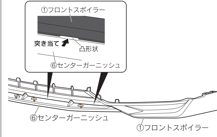
図 17 ※LH図示 左右共通作業
