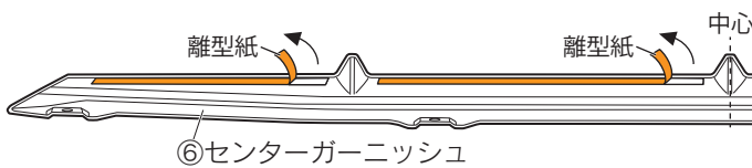
図 16 下面視 ※LH図示 左右共通作業
