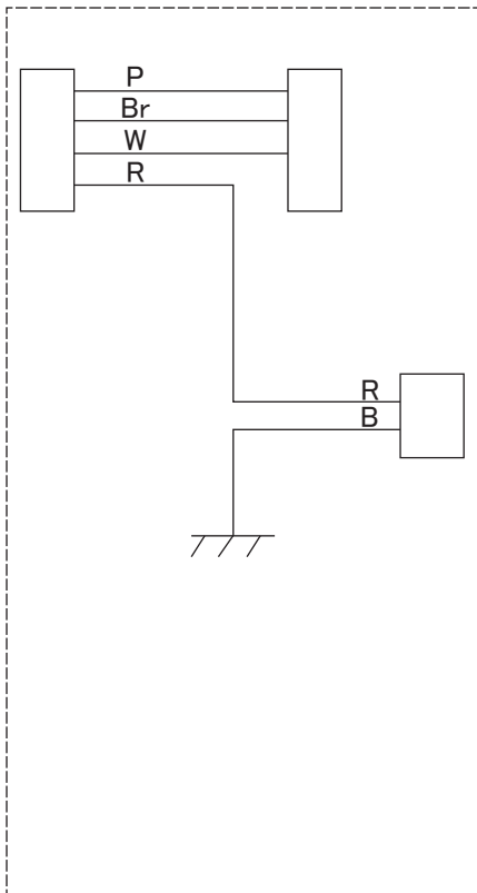
接続ハーネス(車両側)
