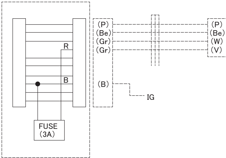
接続ハーネス(車両側)
