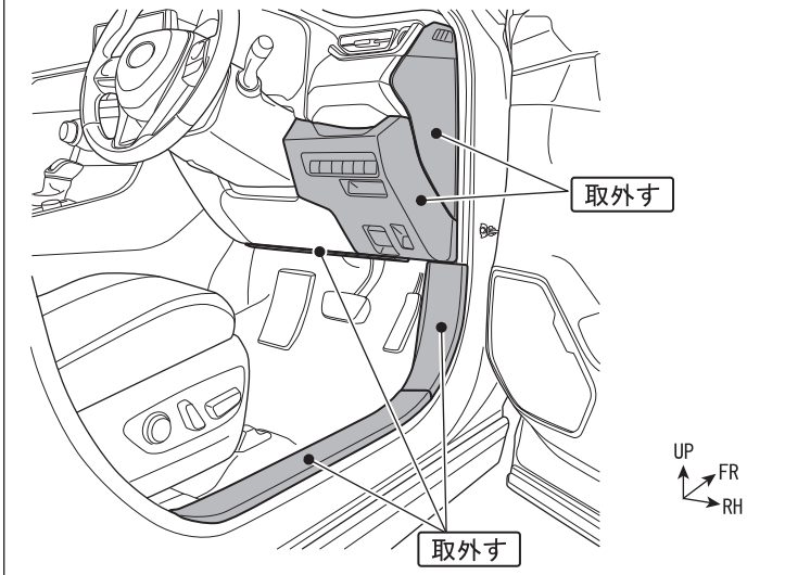
図7 [室内運転席側]
