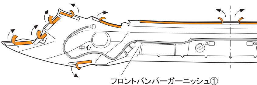
図 16 裏面視 ※LH図示 左右共通作業
