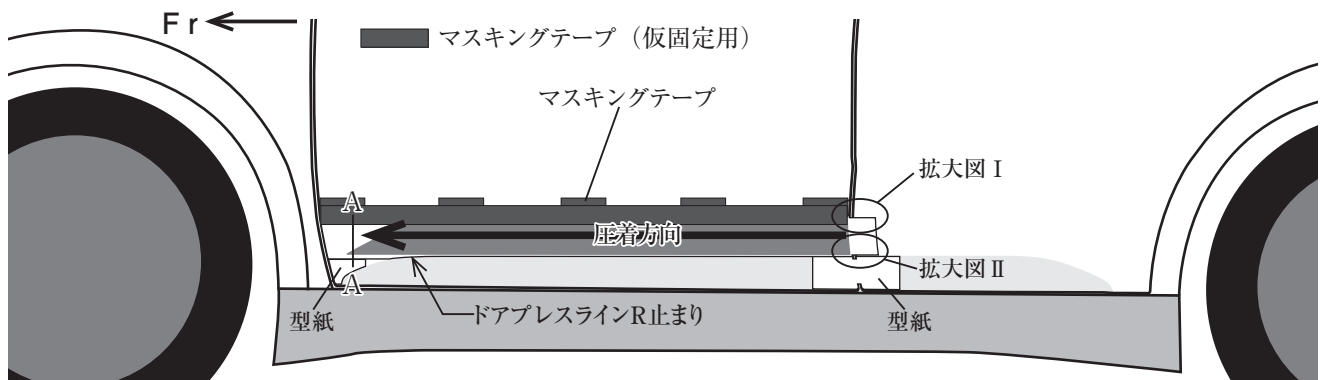
図1 LHFr ドア図
