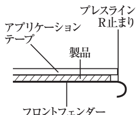
B-B断面図
