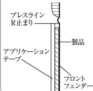
C-C断面図
