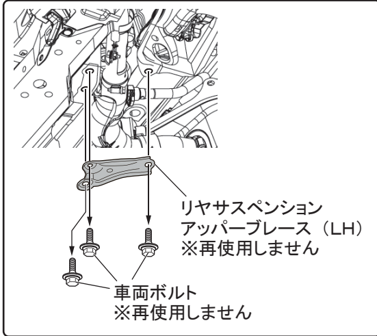
図4 下面視
