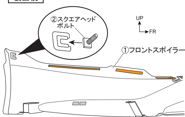
図6 裏面視 ※LH図示 左右共通作業
