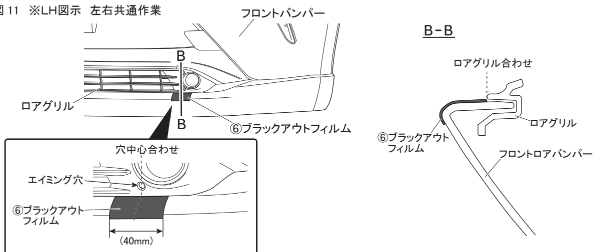
図 11 ※LH図示 左右共通作業
