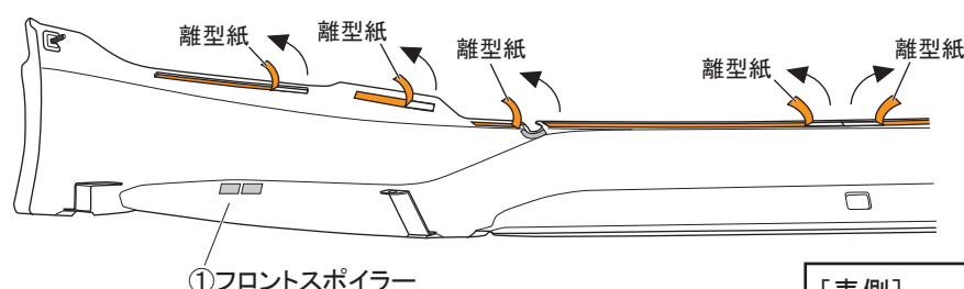
図 12 裏面視 ※LH図示 左右共通作業
