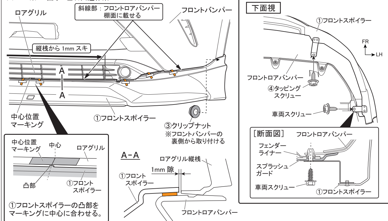
図 13 ※LH図示 左右共通作業
