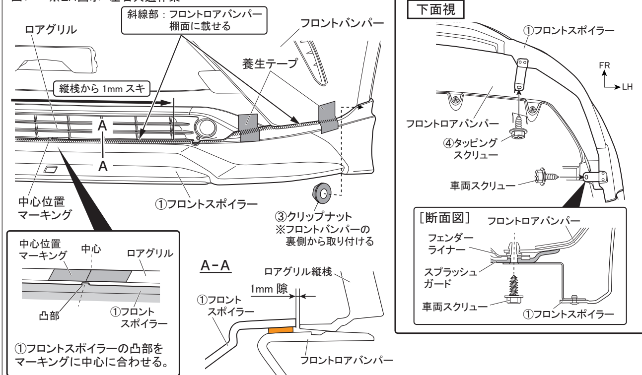
図7 ※LH図示 左右共通作業
