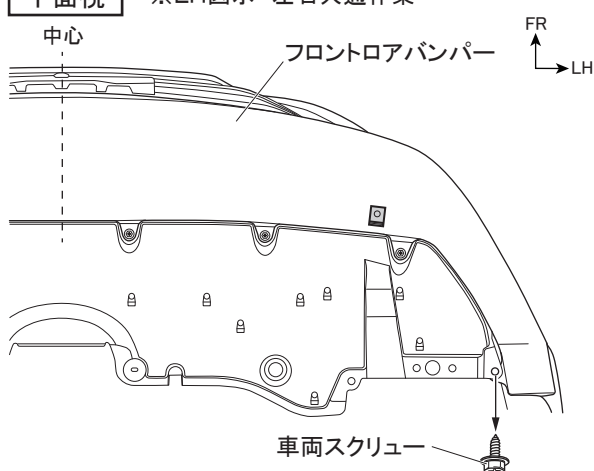
図4 下面視 ※LH図示 左右共通作業
