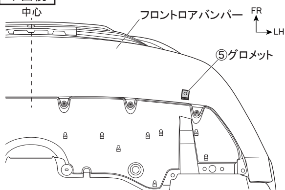
図3 下面視 ※LH図示 左右共通作業
