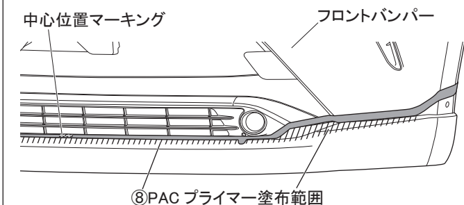
図 10 ※LH図示 左右共通作業
