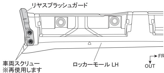
図1 下面視 ※LH図示 左右共通作業
