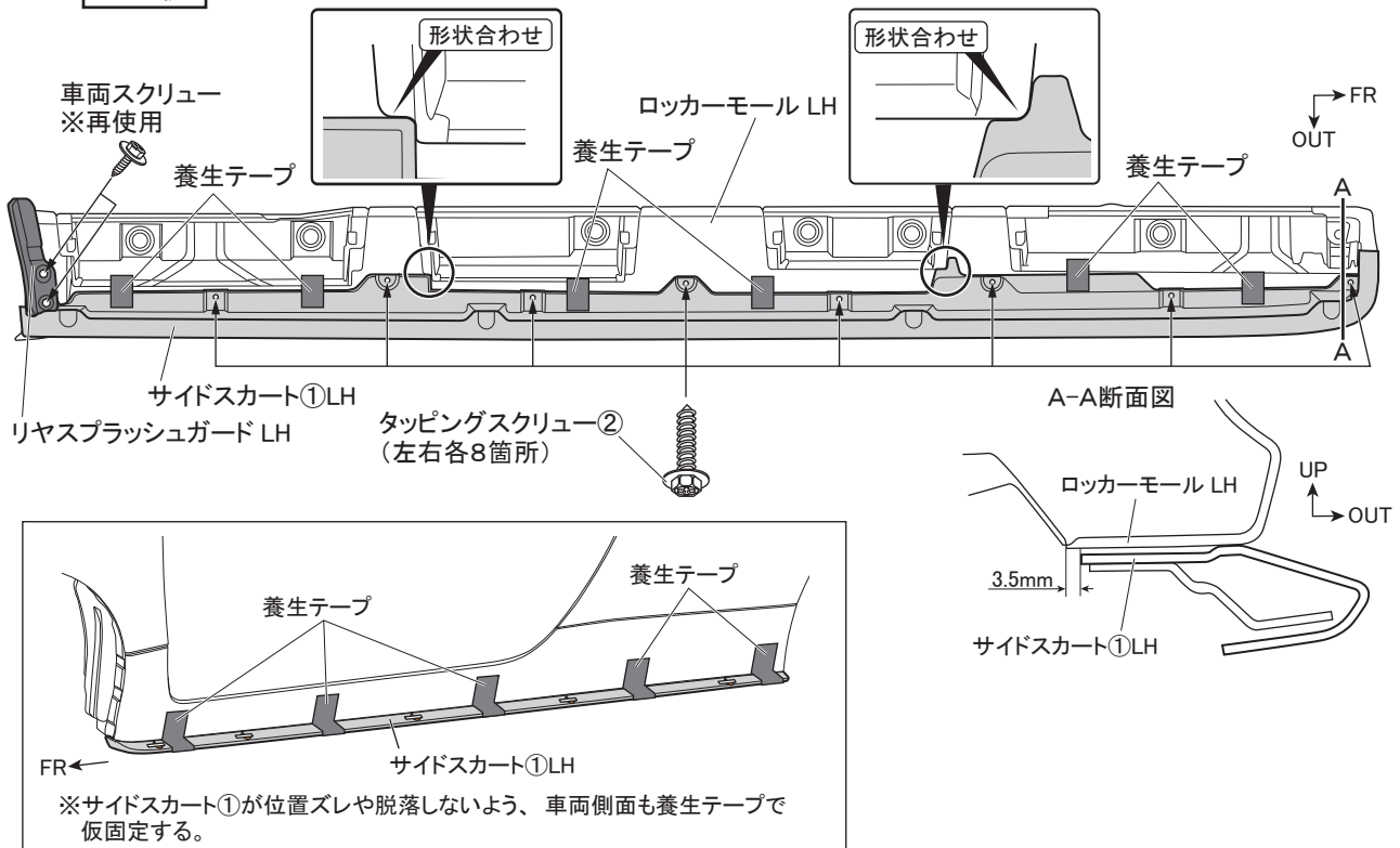
図 10 下面視 ※LH図示 左右共通作業
