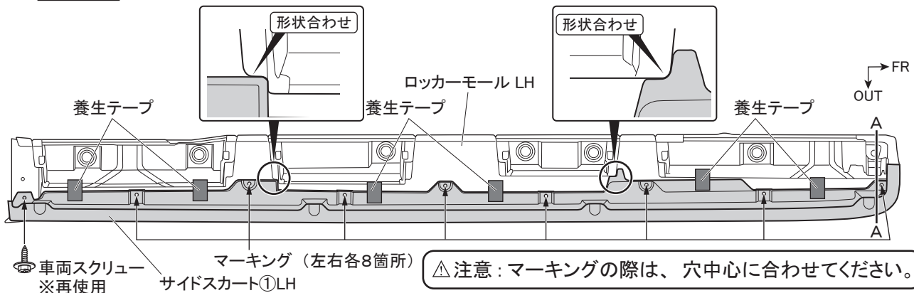
図2 下面視 ※LH図示 左右共通作業
