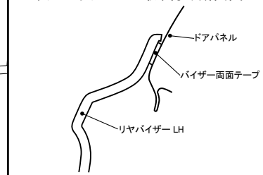
リアバイザー LH 取り付け断面図
