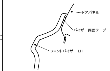
フロントバイザー LH 取り付け断面図
