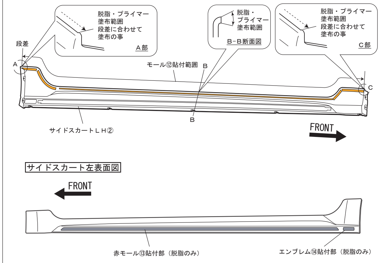
図2 サイドスカート左裏面図
