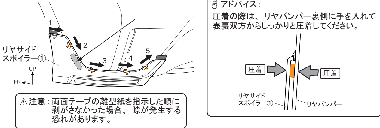
図 25 ※LH図示 左右共通作業
