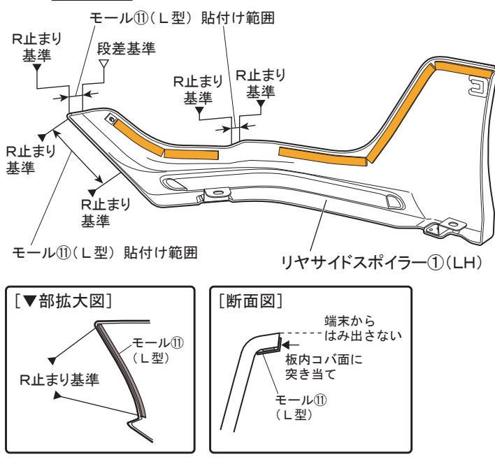
図5 裏面視 ※LH図示 左右共通作業
