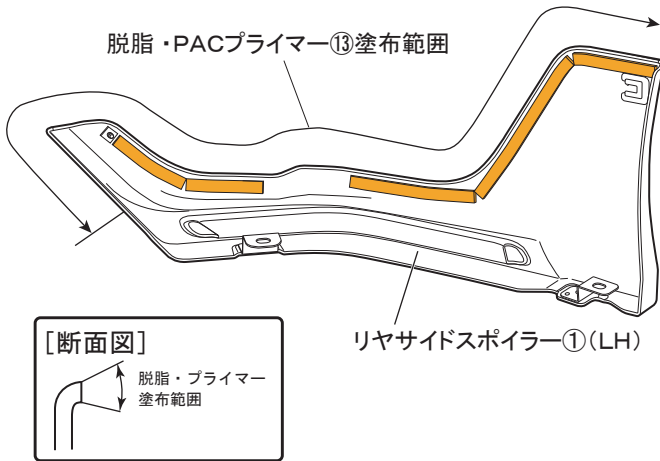
図3 裏面視 ※LH図示 左右共通作業
