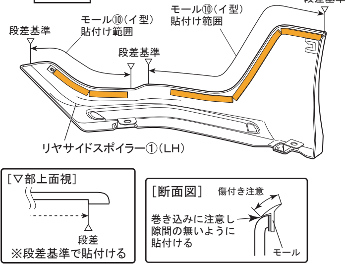
図4 裏面視 ※LH図示 左右共通作業
