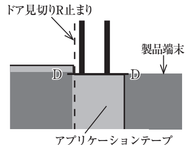
拡大図 IV
