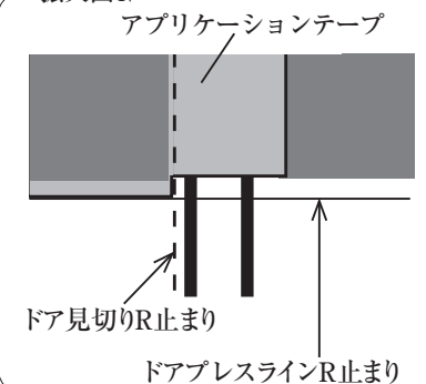
拡大図 IV
