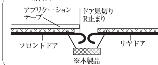
D-D 断面図
