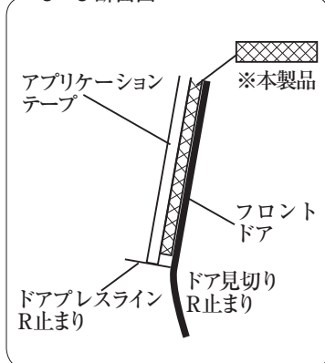
C-C 断面図
