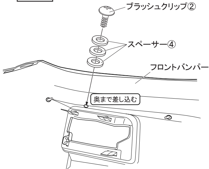
図10 裏面視 ※LH図示 左右共通作業
