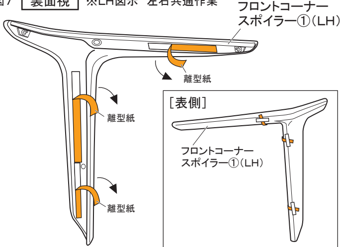
図7 裏面視 ※LH図示 左右共通作業
