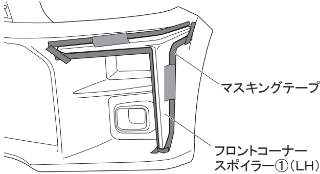
図4 ※LH図示 左右共通作業
