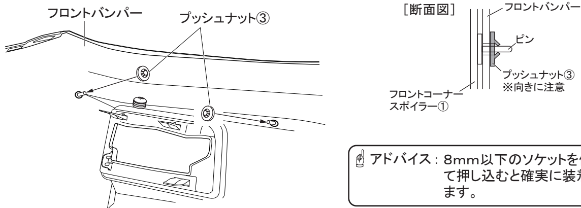
図 12 裏面視 ※LH図示 左右共通作業
