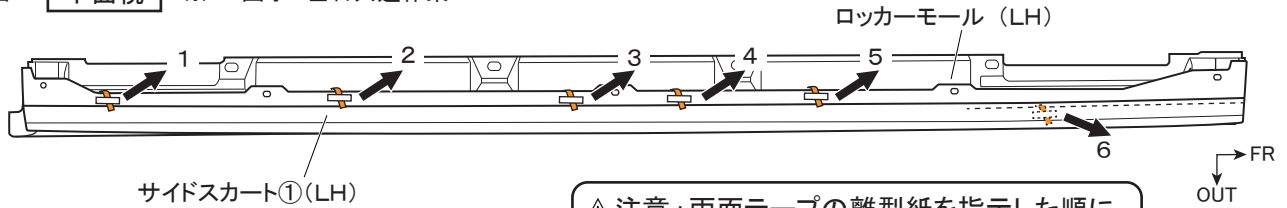
図9 下面視 ※LH図示 左右共通作業
