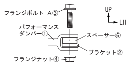
[締結部断面図 LH]
