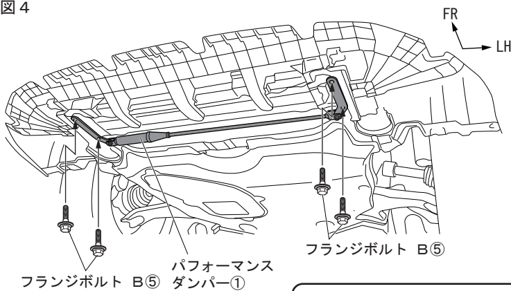
[下面視]
