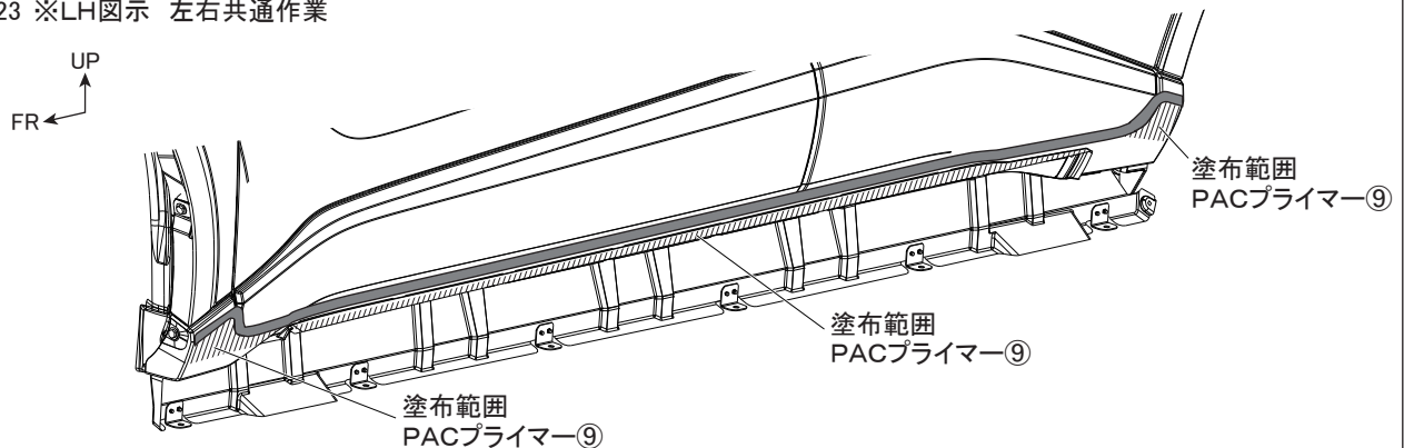
図 23 ※LH図示 左右共通作業
