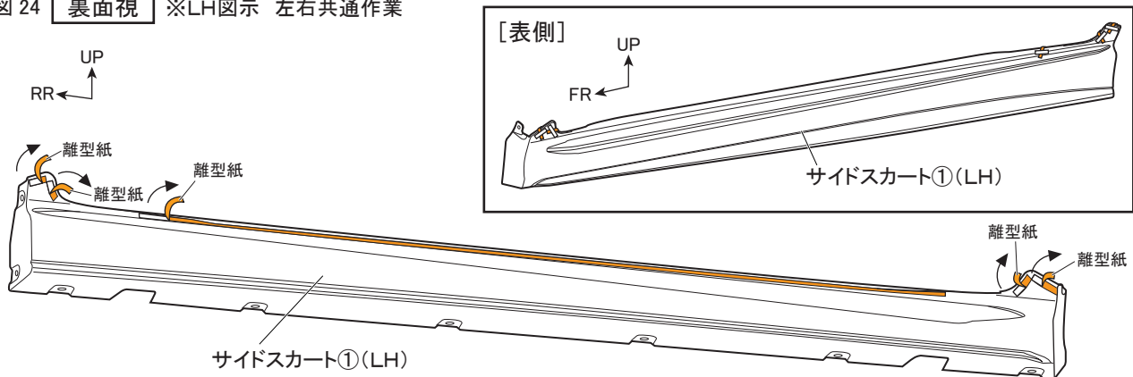
図 24 裏面視 ※LH図示 左右共通作業
