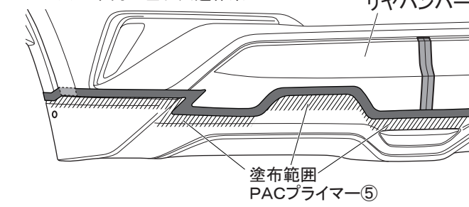
図 14 ※LH図示 左右共通作業
