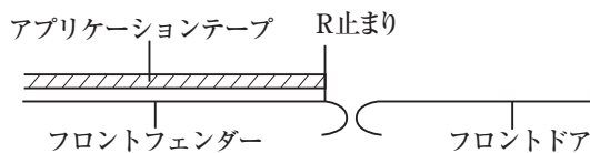
A-A 断面図
