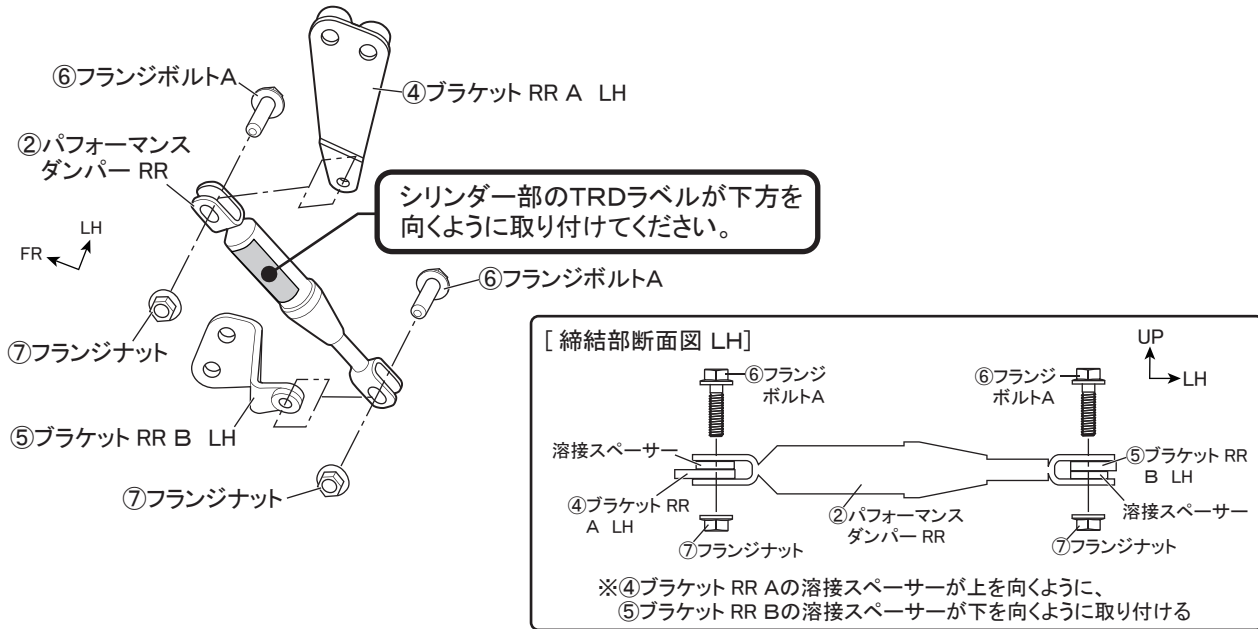
図7 下面視 ※LH図示 左右共通作業
