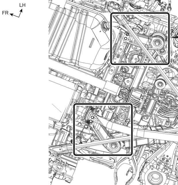
図10 下面視 ※図は4WD車、2WD車も共通
