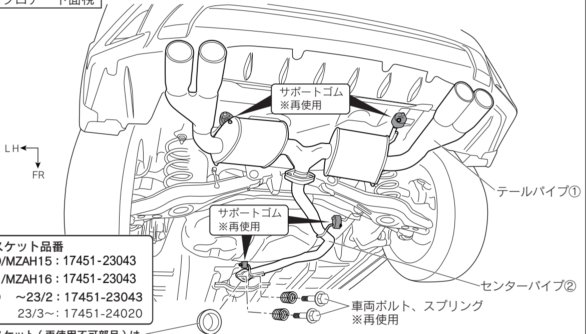
図2 リヤフロアー下面視
