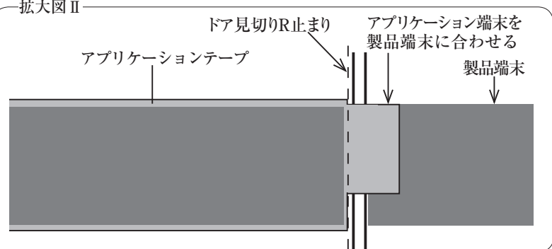
拡大図Ⅱ
