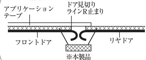
D-D断面図
